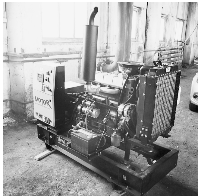
Новый дизель-генератор приобретен по программе «Народный бюджет».
